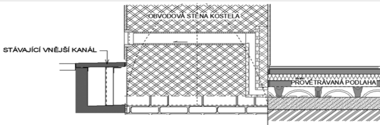
Návaznost provětrávané podlahy na stěnu – svislý řez
